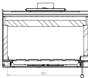
PRZĘKRÓJ A-A SKALA 1 : 7
