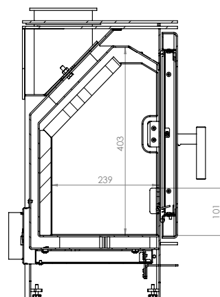
PRZĘKRÓJ B-B SKALA 1 : 7
